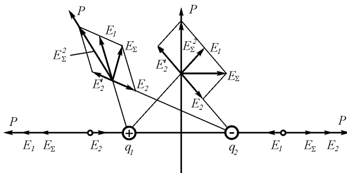
Рис. 7.2. Излучение энергии диполем с сосредоточенными параметрами
