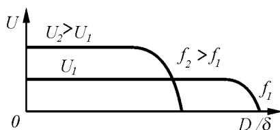
Рис. 7.5. Зависимость сигнала приемника от расстояния между диполями при продольном излучении энергии
