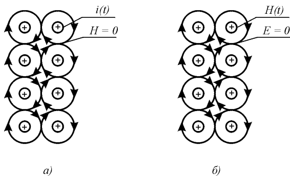
Рис. 5.1. Компенсации полей: a — магнитного поля в распределенной системе токов; б — электрического поля в распределенной системе магнитных потоков
