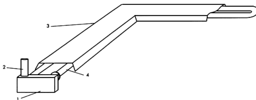
Рисунок Б.3 - Центральный газовоздушный инфракрасный излучатель - "темный":
