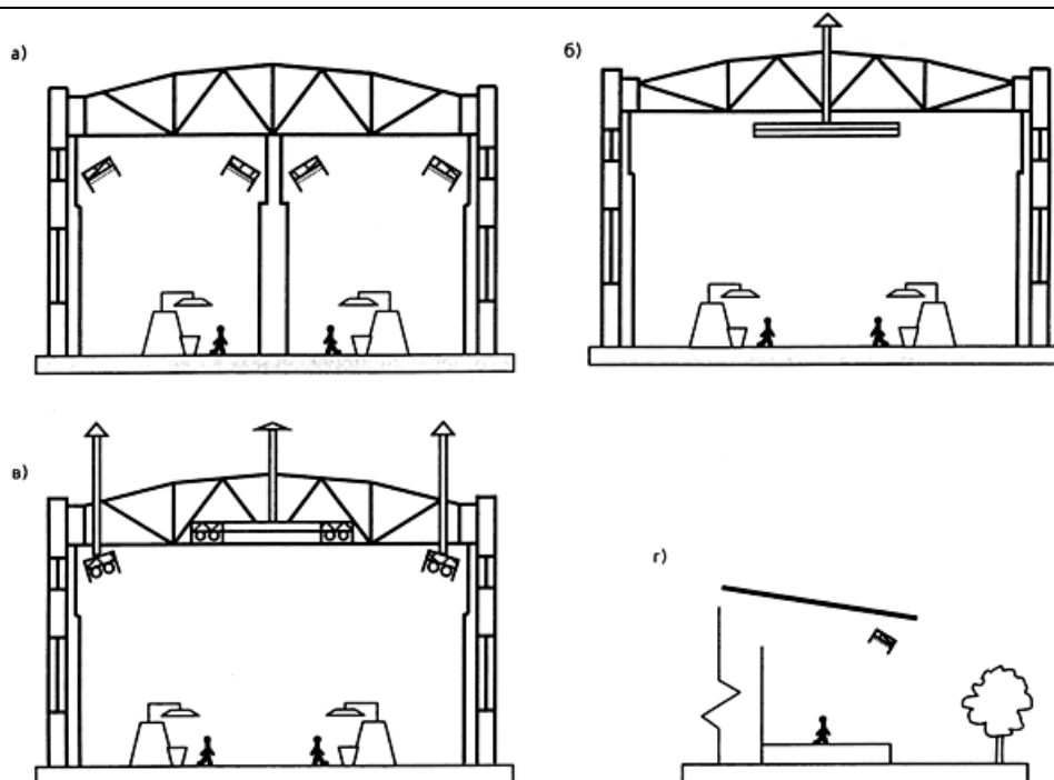
Рисунок 1 - Варианты размещения ГИИ при отоплении помещений и обогреве отдельных зон:
