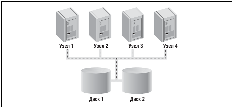
Рис. 9.6. Архитектура RAC
