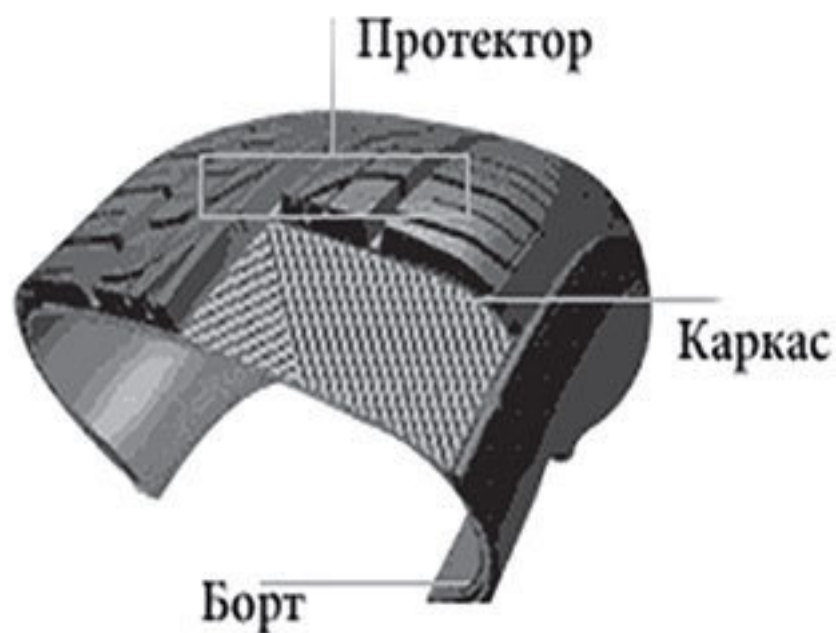
Рис 19. Радиальные и диагональные шины
