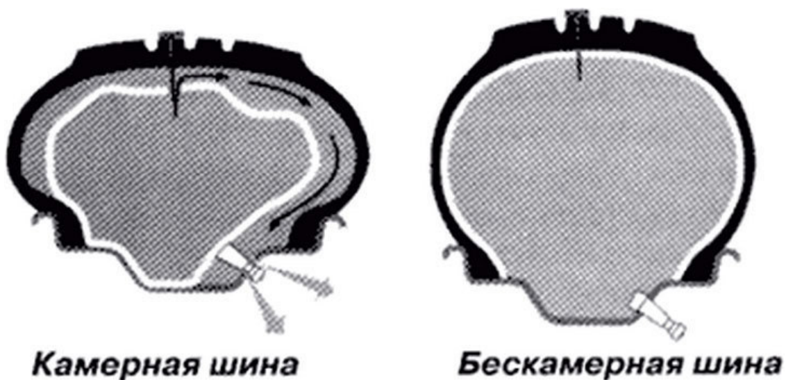
Рис. 33. Сравнительные характеристики камерной и бескамерной шины
