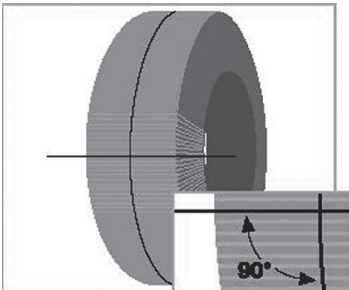
Рис. 20. Расположение нитей корда радиальной шины
