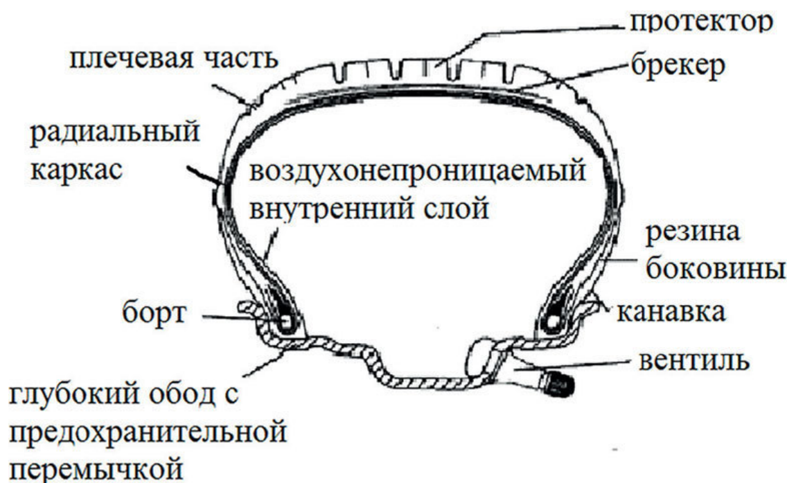
Рис. 25. Устройство бескамерной шины
