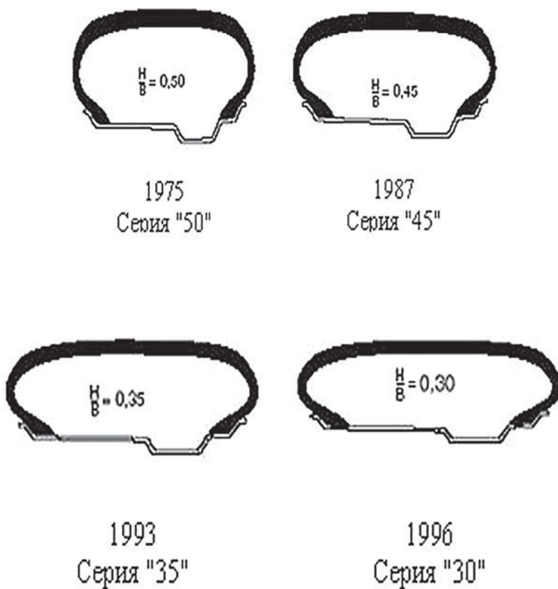
Рис. 22. Изменение профиля пневматической шины с 1975 по 1996 гг.
