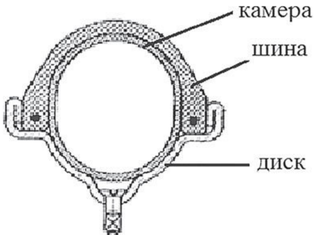
Рис. 24. Камерная шина
