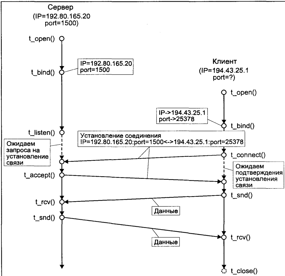
Рис. 6.18. Схема вызова функций ТЛ для протокола с предварительным установлением соединения
