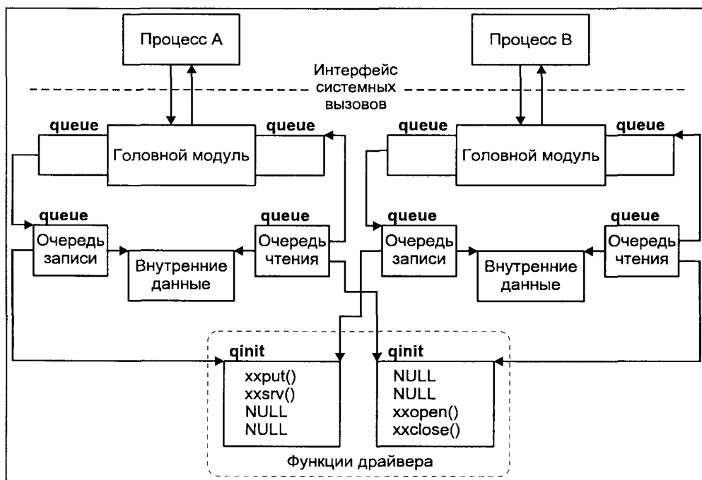
Рис. 5.23. Верхний мультиплексор
