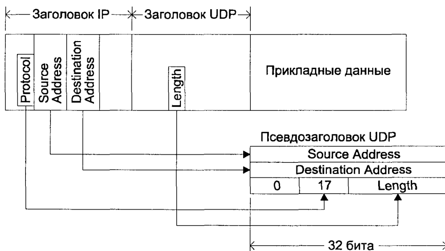
Рис. 6.10. Псевдозаголовок UDP
