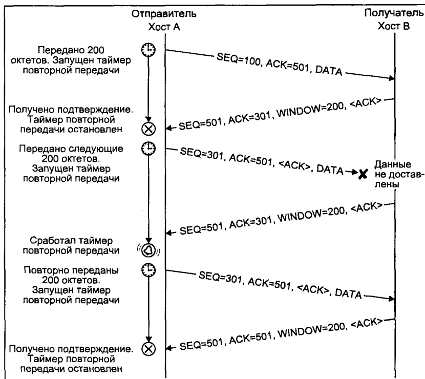
Рис. 6.13. Повторная передача
