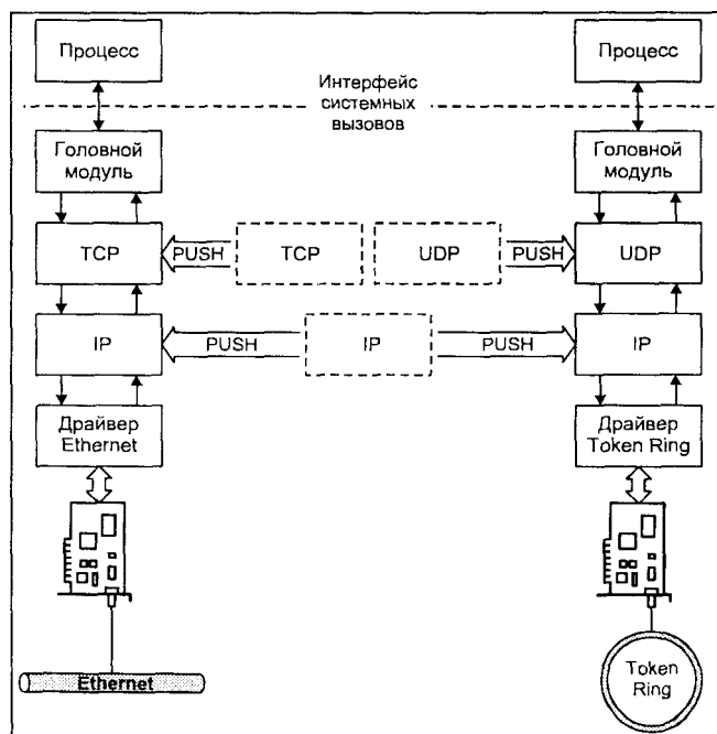
Рис. 5.14. Использование одних и тех же модулей для создания различных потоков
