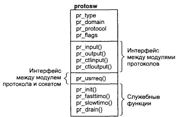
Рис. 6.22. Коммутатор протокола
