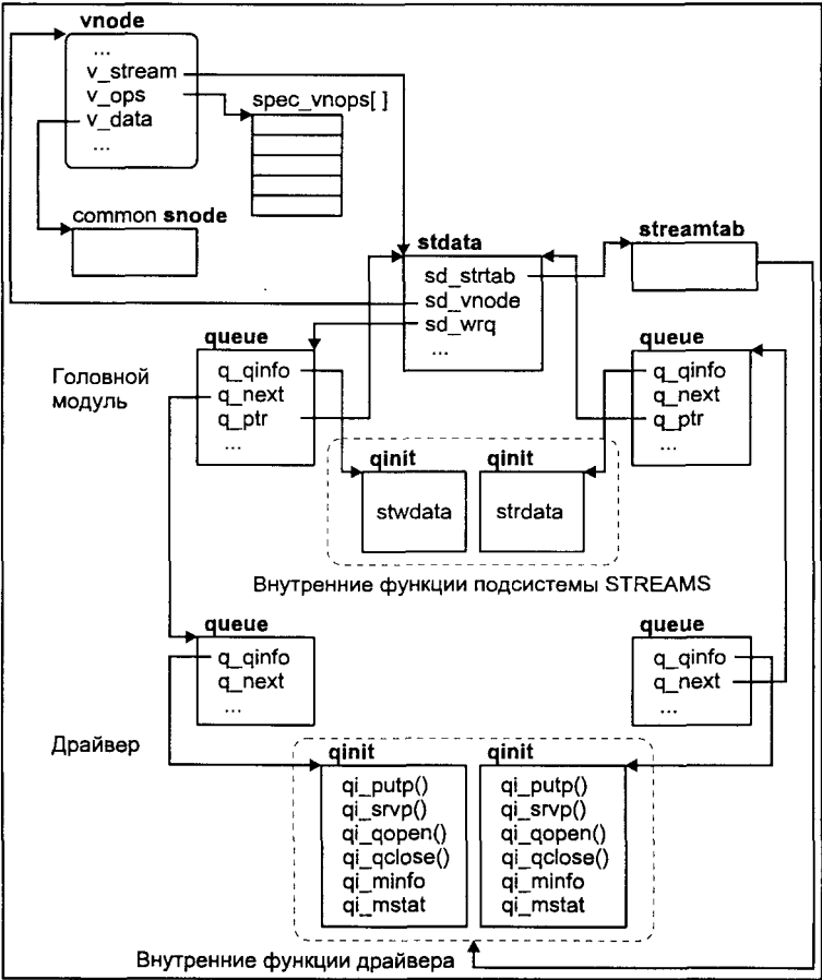
Рис. 5.22. Структура потока после открытия
