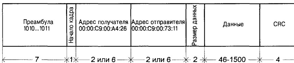
Рис. 6.37. Формат кадра IEEE 802.3
