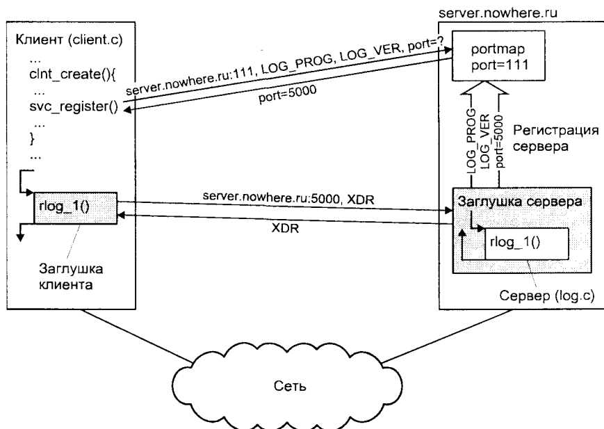
Рис. 6.20. Работа системы RPC
