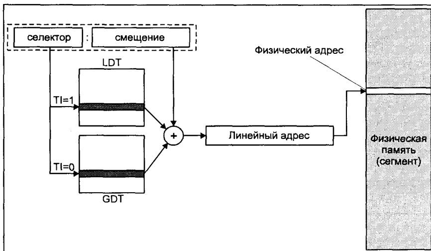
Рис. 3.6. Трансляция адреса с использованием механизма сегментации
