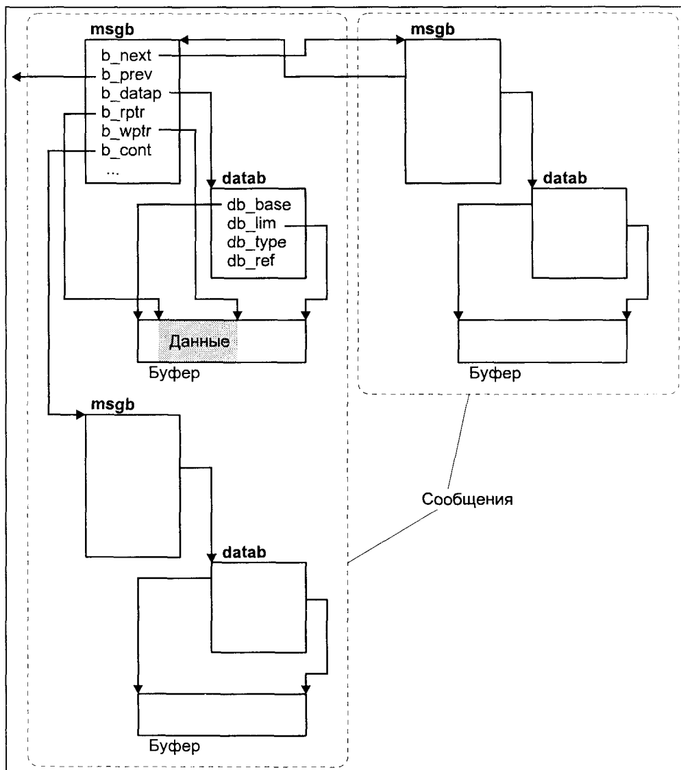
Рис. 5.17. Сообщения STREAMS
