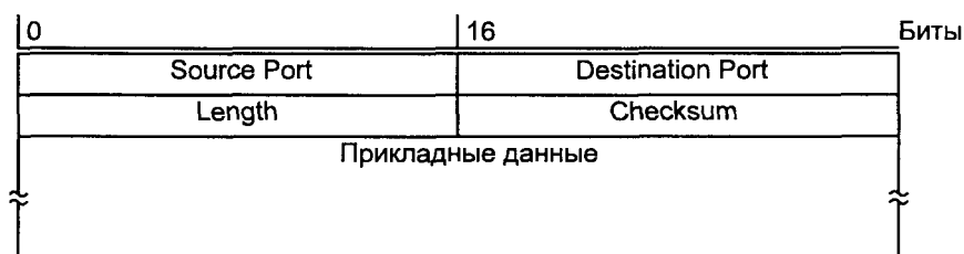
Рис. 6.9. Заголовок UDP
