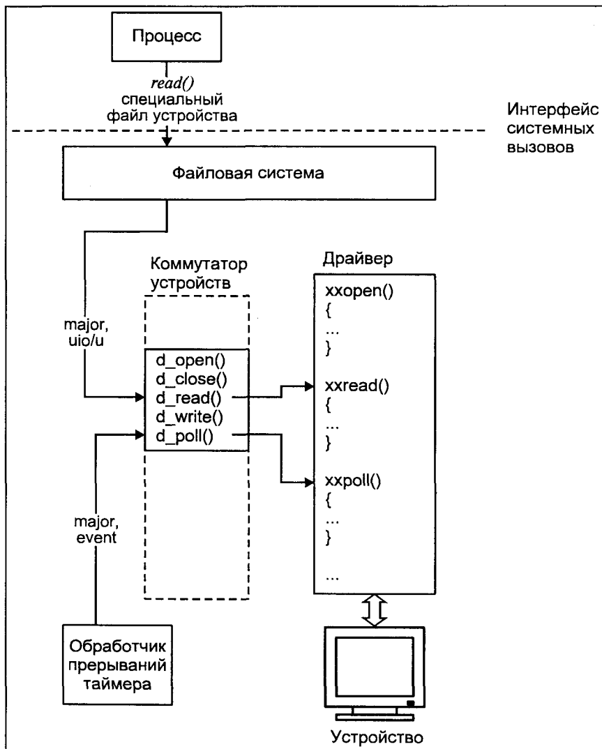
Рис. 5.2. Доступ к драйверу символического устройства
