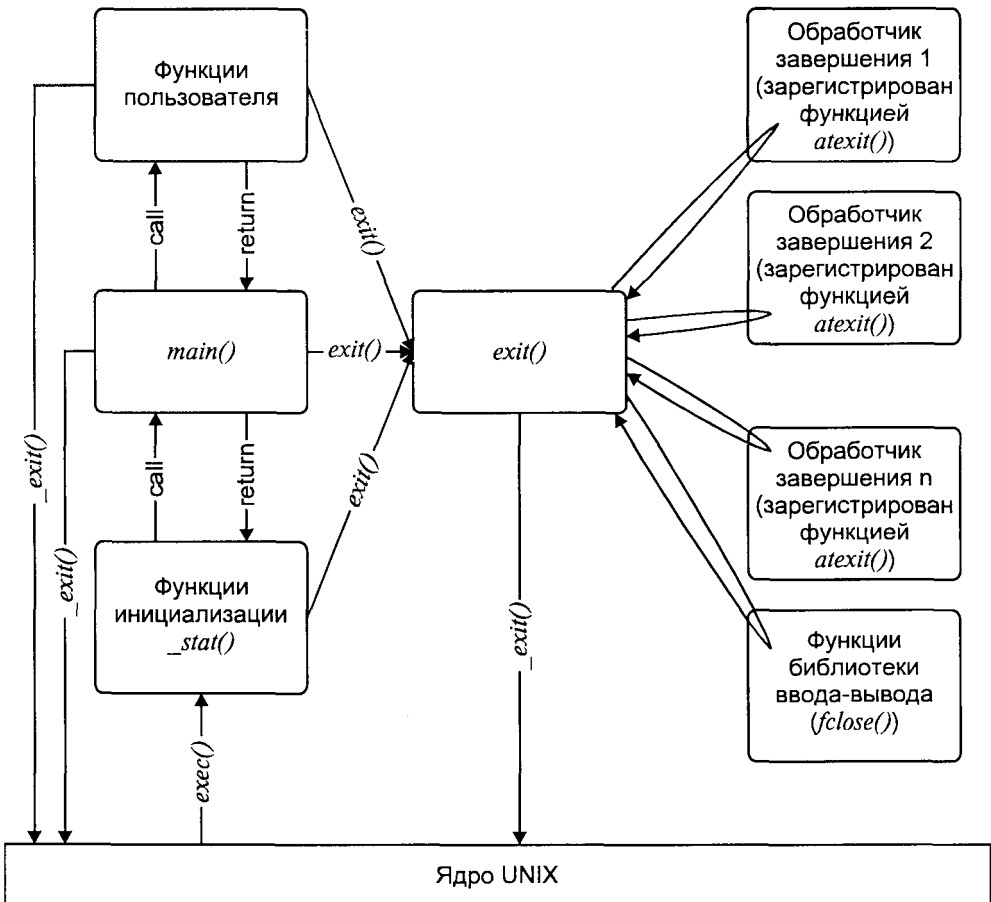
Рис. 2.7. Запуск и завершение C-программы
