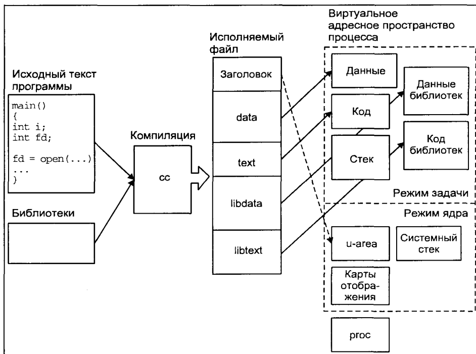
Рис. 3.1. Инфраструктура процесса операционной системы UNIX
