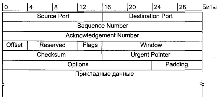
Рис. 6.11. Формат TCP-сегмента
