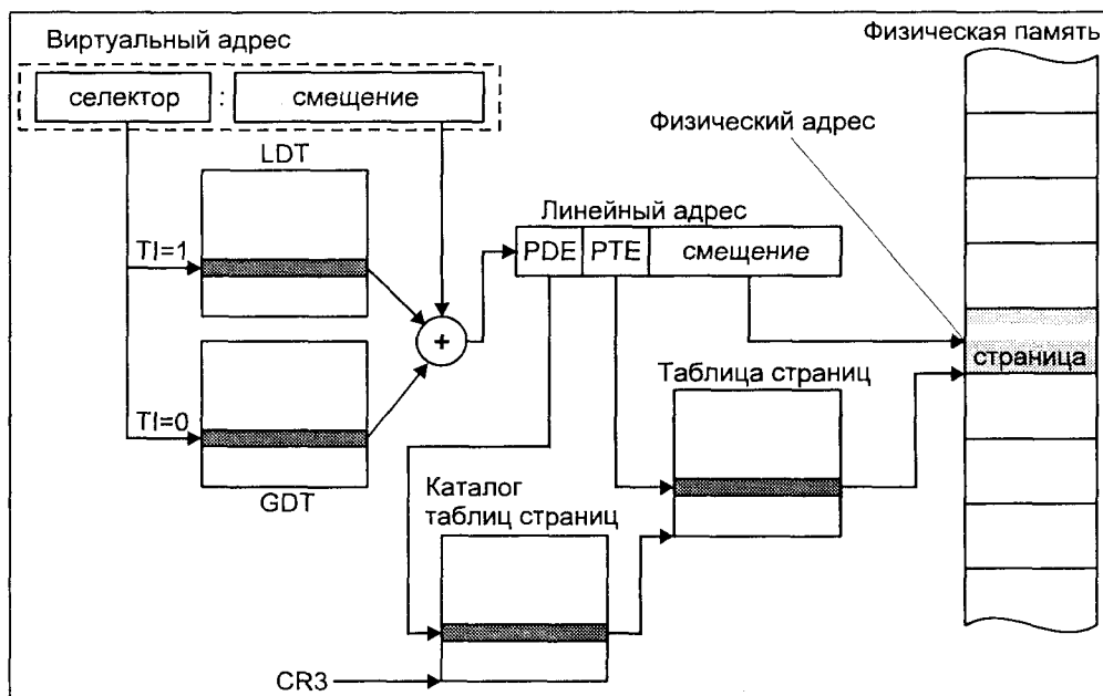
Рис. 3.7. Трансляция адреса с использованием страничного механизма
