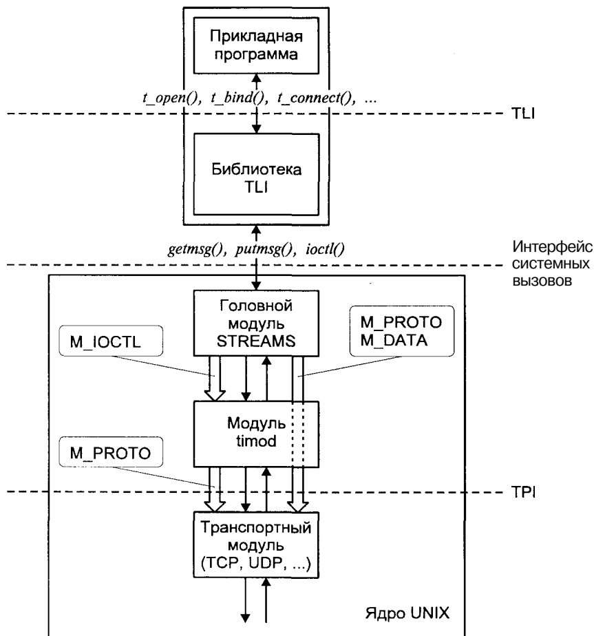
Рис. 6.33. Архитектура доступа к транспортным услугам
