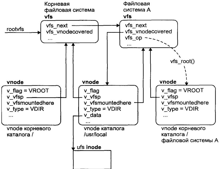
Рис. 4.11. Схема монтирования файловых систем различных типов
