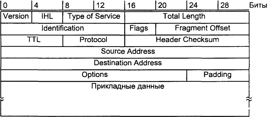
Рис. 6.6. Заголовок IP-датаграммы
