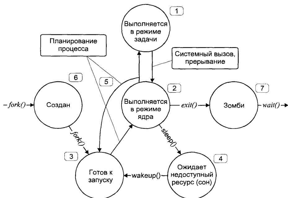
Рис. 3.3. Состояния процесса
