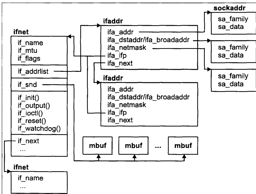
Рис. 6.23. Сетевой интерфейс
