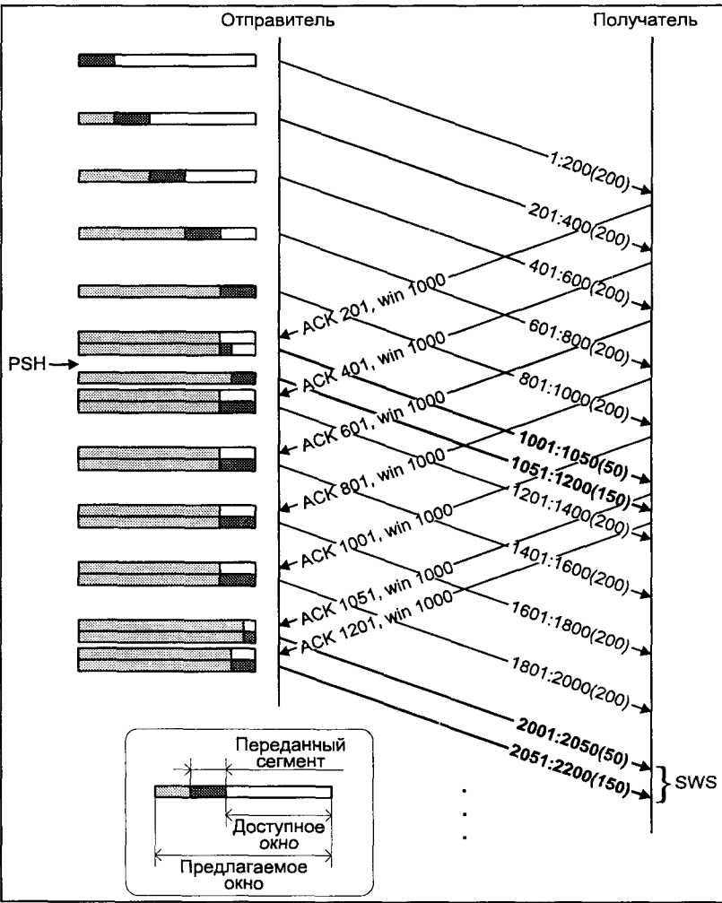
Рис. 6.15. Возникновение SWS
